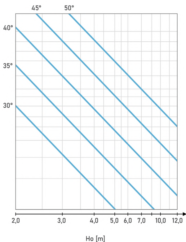
NWO-12 ( \phi 315 ) ogrzewanie
