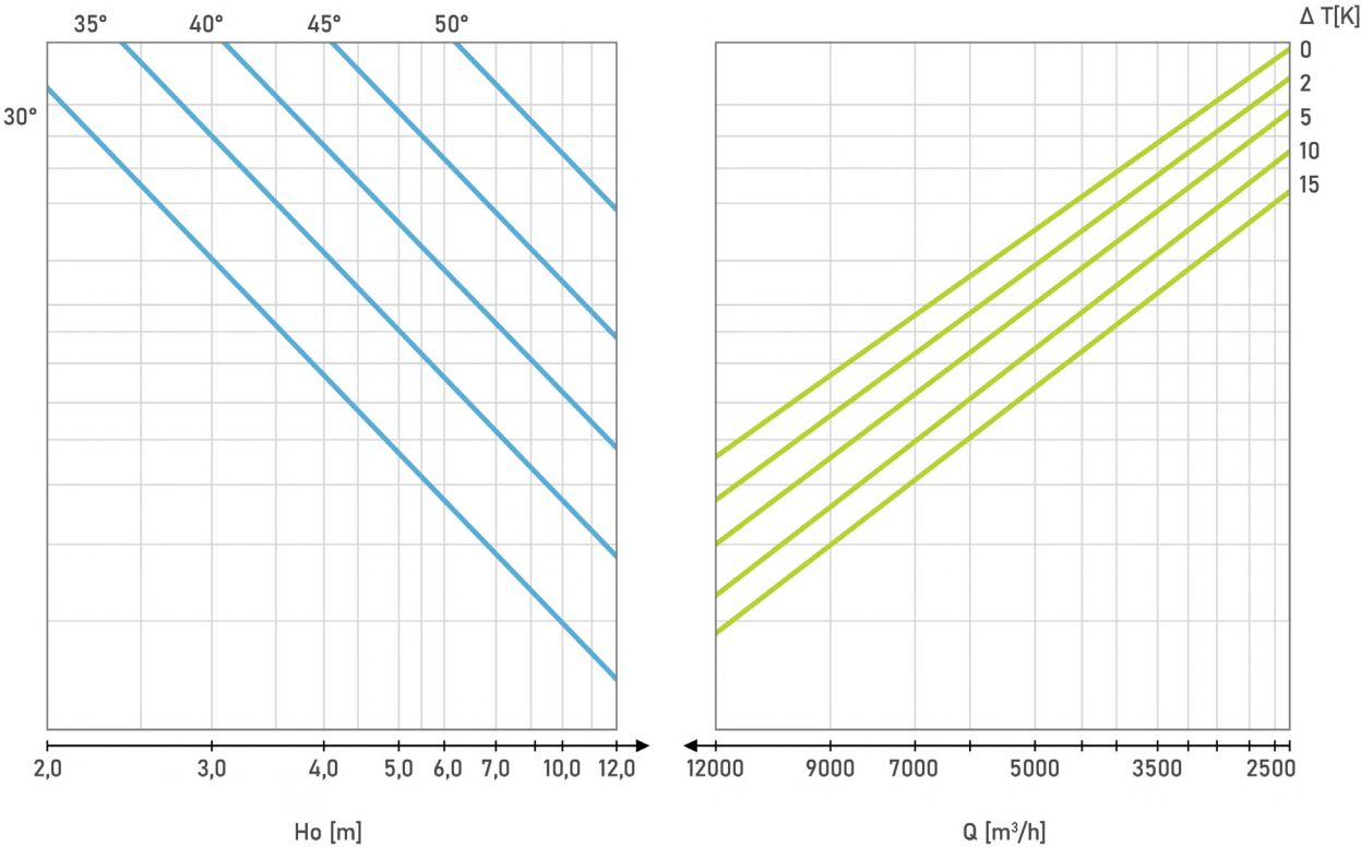
NWO-12 (φ800) ogrzewanie
