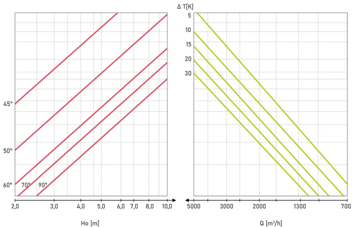
NWO-12 (φ500) ogrzewanie
