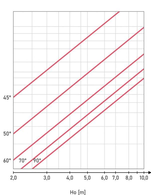
NWO-12 ( \phi 400 ) ogrzewanie
