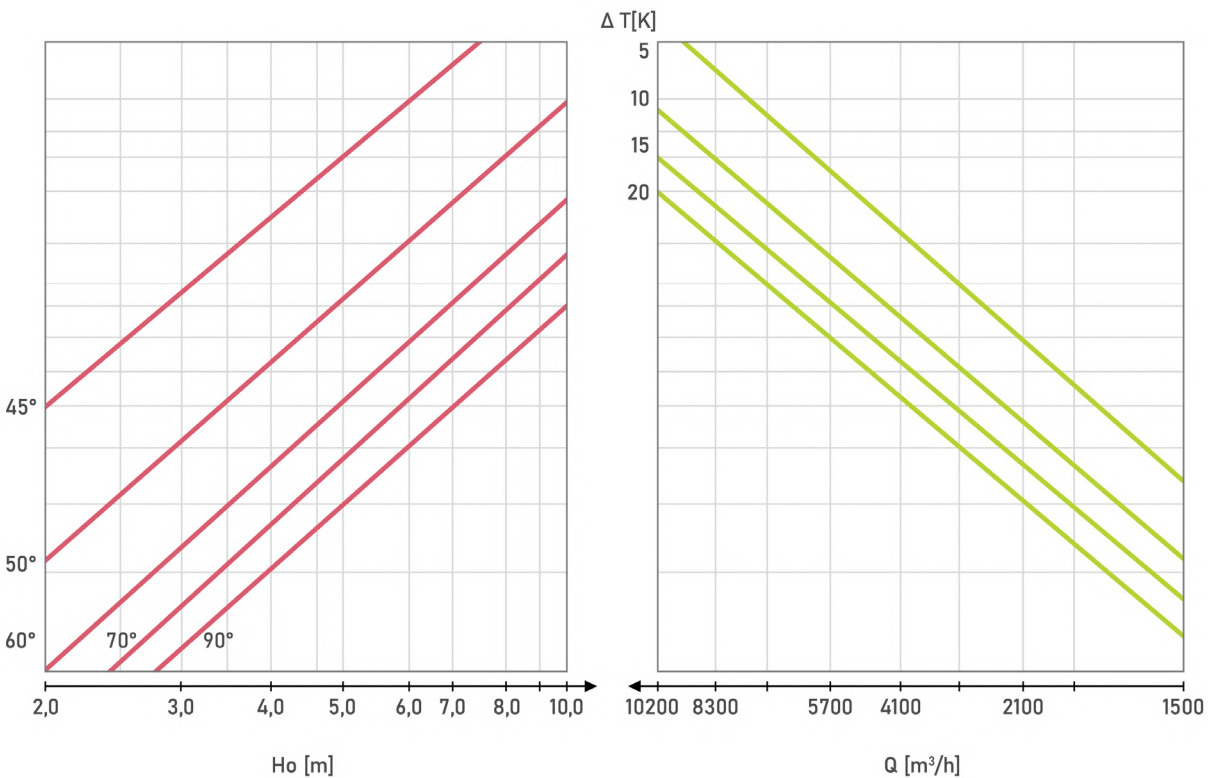
NWO-12 (φ710) ogrzewanie
