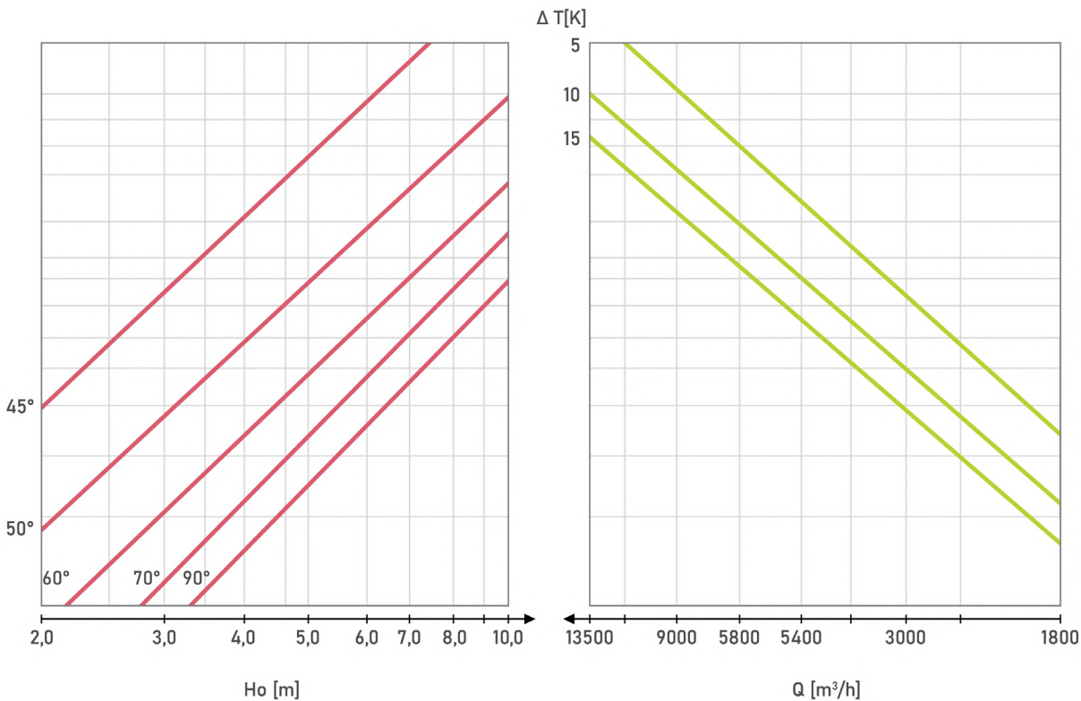
NWO-12 (φ800) ogrzewanie
