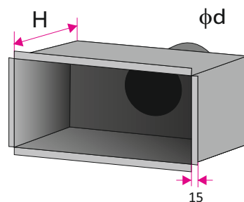
SR-Tw - Skrzynka rozprężna z króćcem tylnym
