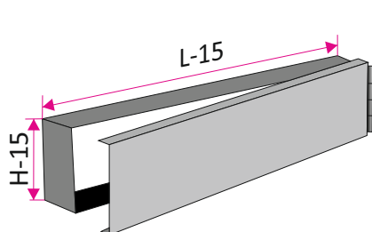
GU - przepustnica uchylna (szczególnie zalecana do kratki na kanał spiro)
