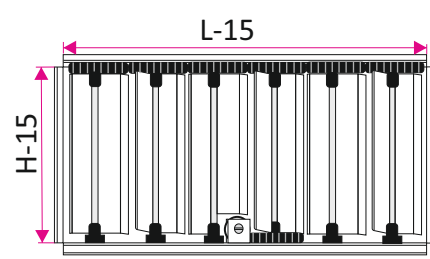
GP - przepustnica przeciwbieżna (powyżej wielkości 525x425 przepustnica jest dzielona)
