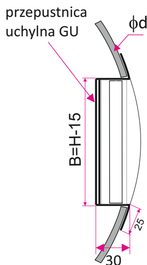
L,H - wymiary otworu montażowego kratki
