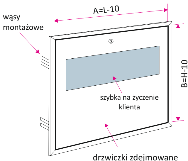
Przykładowe wymiary szafek
